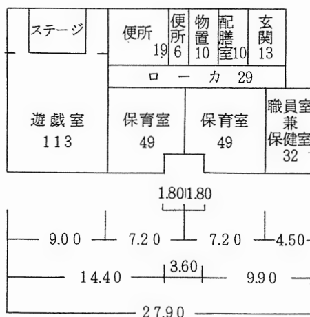
すがま幼稚園平面図
