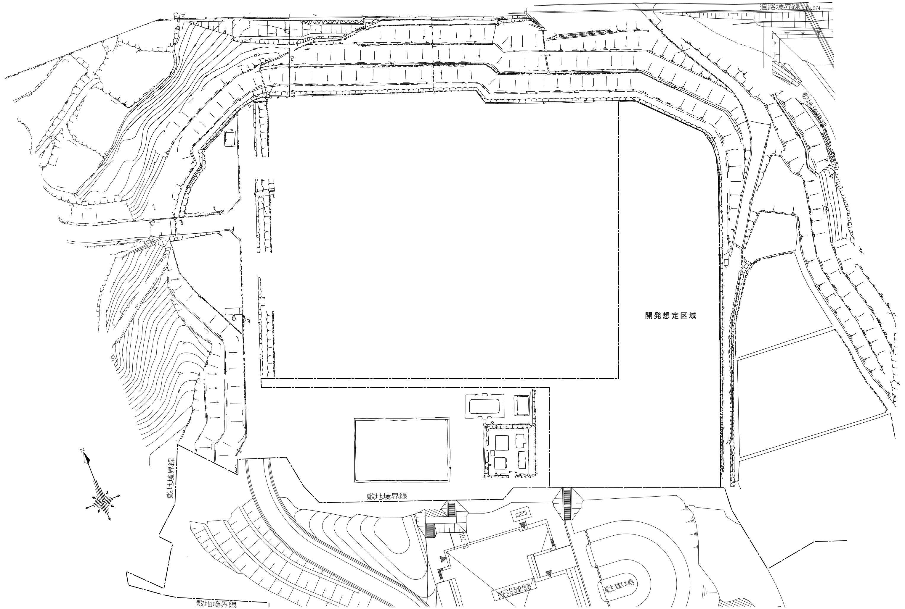
開発想定区域図 S=1:1000
