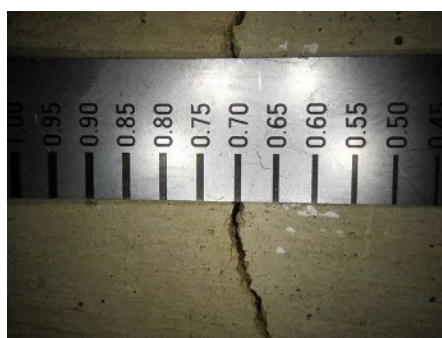
38. 兎田橋：鋼I桁橋 (橋長：23.40m、1994年竣工) 橋台前面の鉛直方向ひびわれ ※雨水の浸入により、損傷は進行する可 能性がある。(迂回路有り)
