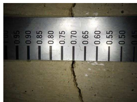
38. 兎田橋：鋼I桁橋 (橋長：23.40m、1994年竣工) 橋台前面の鉛直方向ひびわれ ※雨水の浸入により、損傷は進行する可 能性がある。(迂回路有り)
